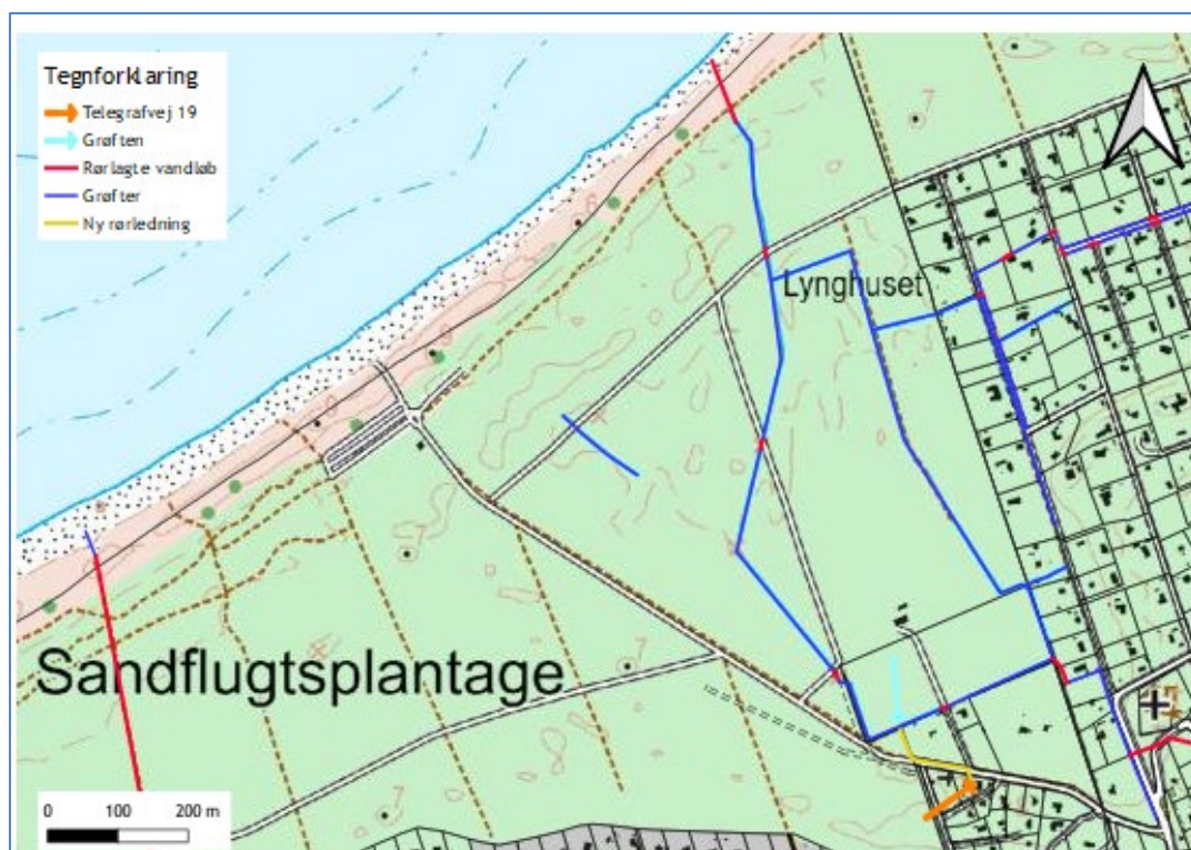
Figur 3 – Grøftens forløb.
