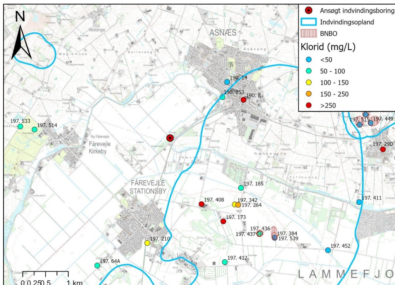
Figur 5b - Kloridkoncentrationer i nærliggende borer
