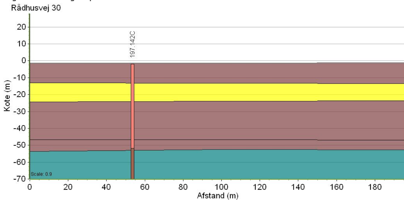
Figur 3b. Lertykkelse over Sand 3
