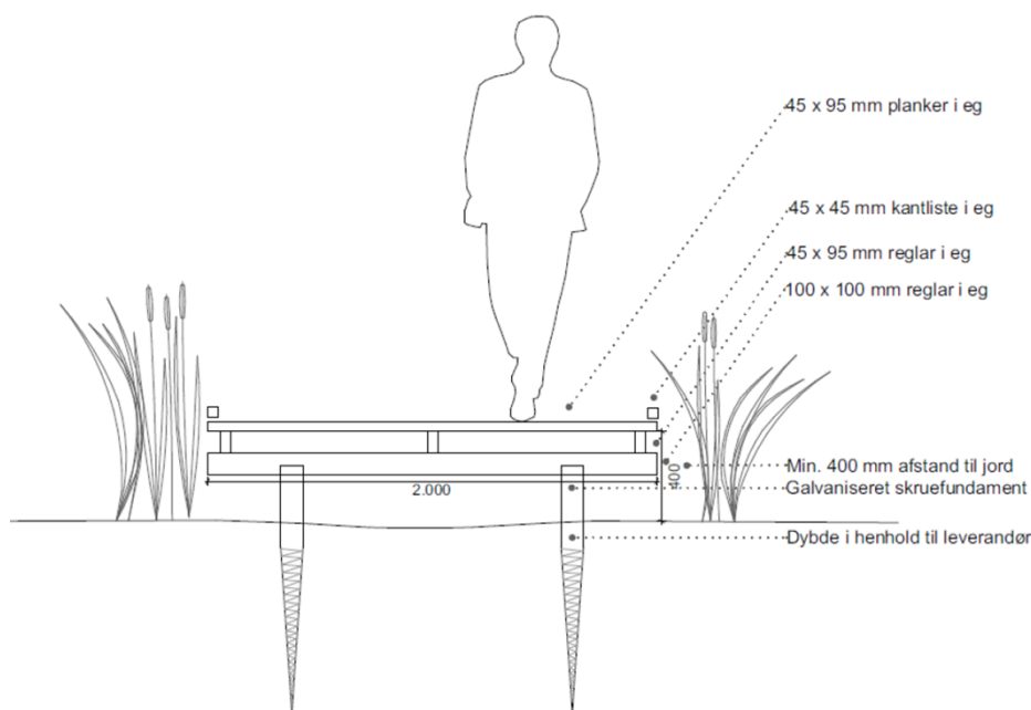
Principsnit af boardwalk over vådområde. (Udklip fra ansøgningen)
