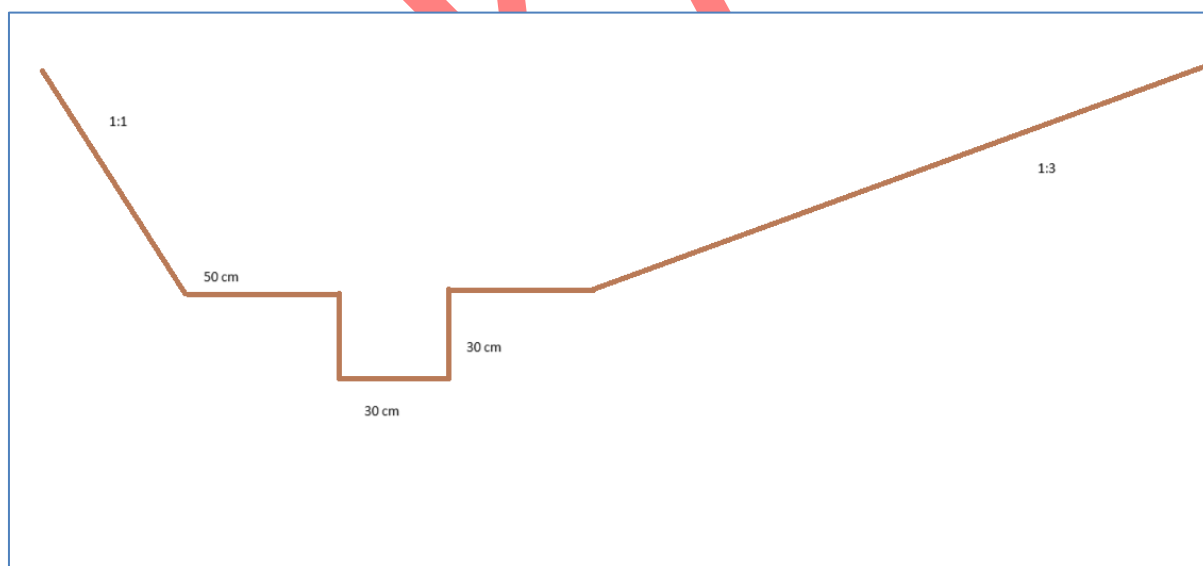
Figur 2: Principskitse dobbeltprofil.
