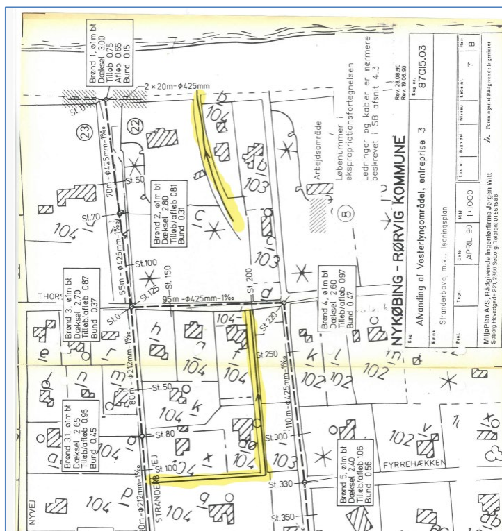
Figur 3 - Anlægstegning Afvanding Vesterlyng 1990. Grøften mellem Stranderbovej og Thorsvej er markeret med gult. De nye afvandsledninger er vist med stiplede sorte linjer.
