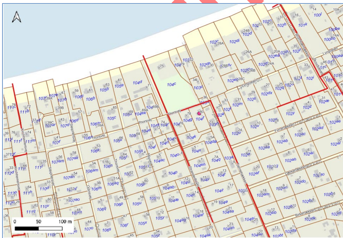
Figur 2 - Afvandingsystem Vesterlyng. Rørledninger er vist med rødt. Thorsvej 80 er markeret med pink prik.
