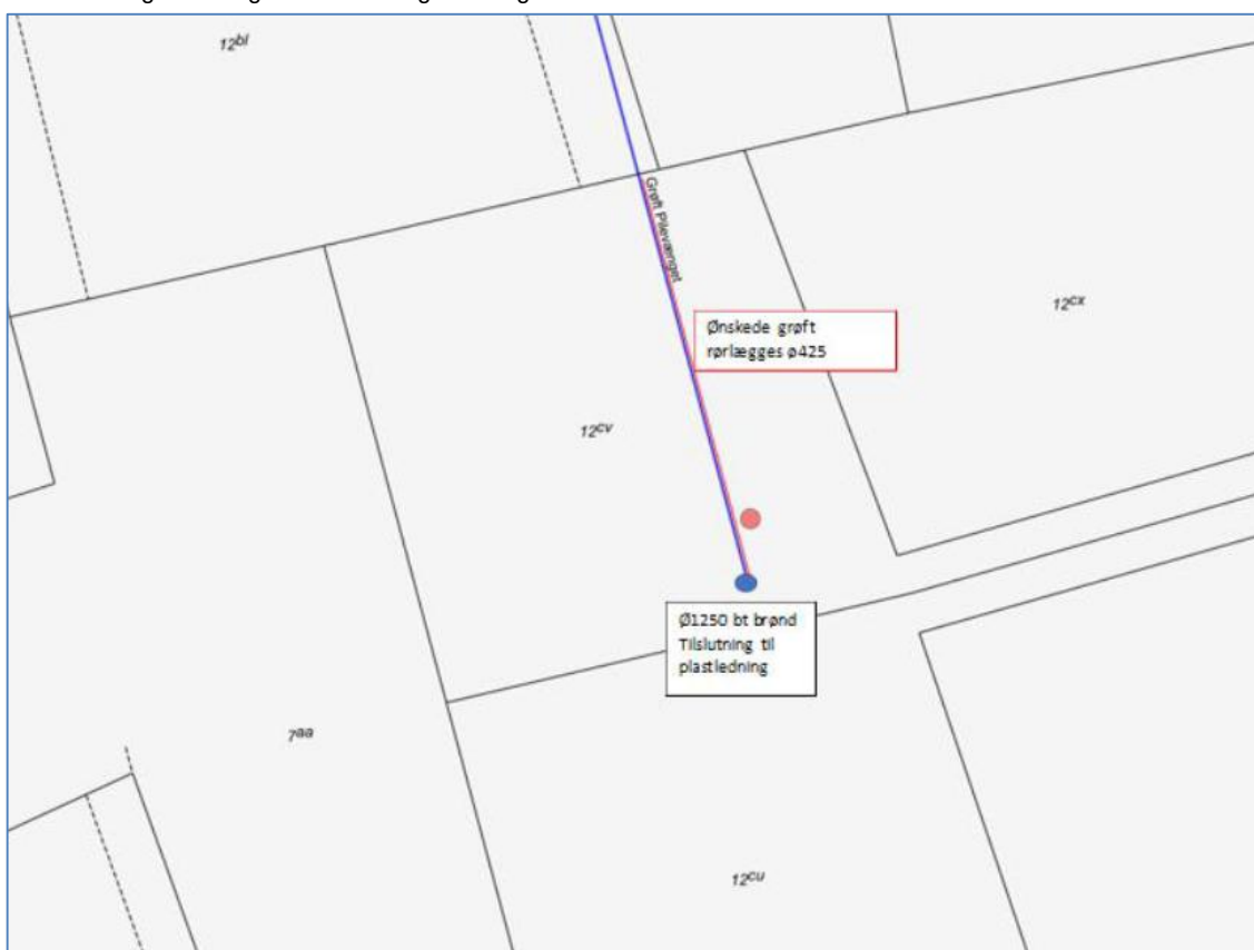
Figur 1. Plantegning fra ansøgningen.
