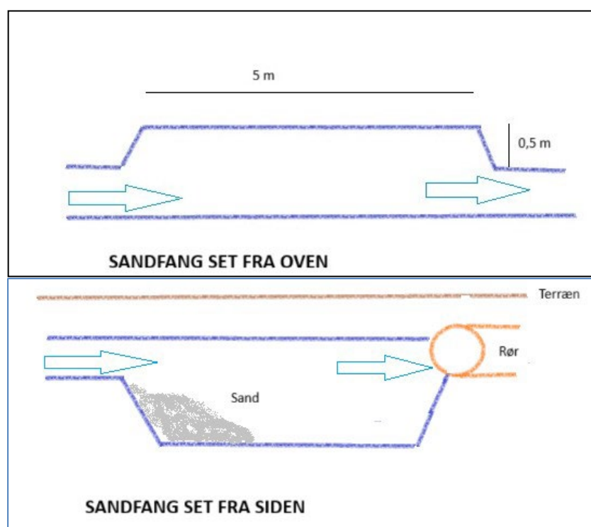
Figur 2 – Principskitser af sandfanget.
