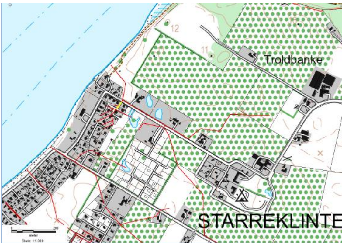
Figur 2 – Dræn er vist med rødt. Projektstrækningen er markeret med gult. Målestok 1:5.000.
