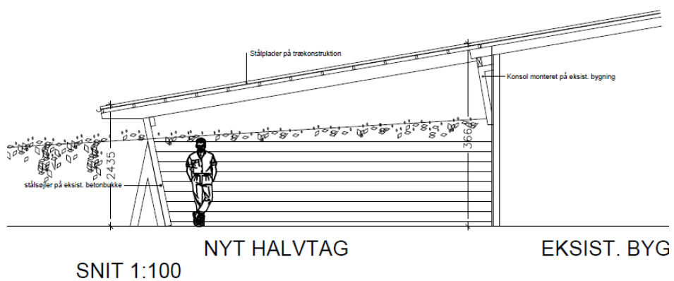
Snittegning fra ansøgning
