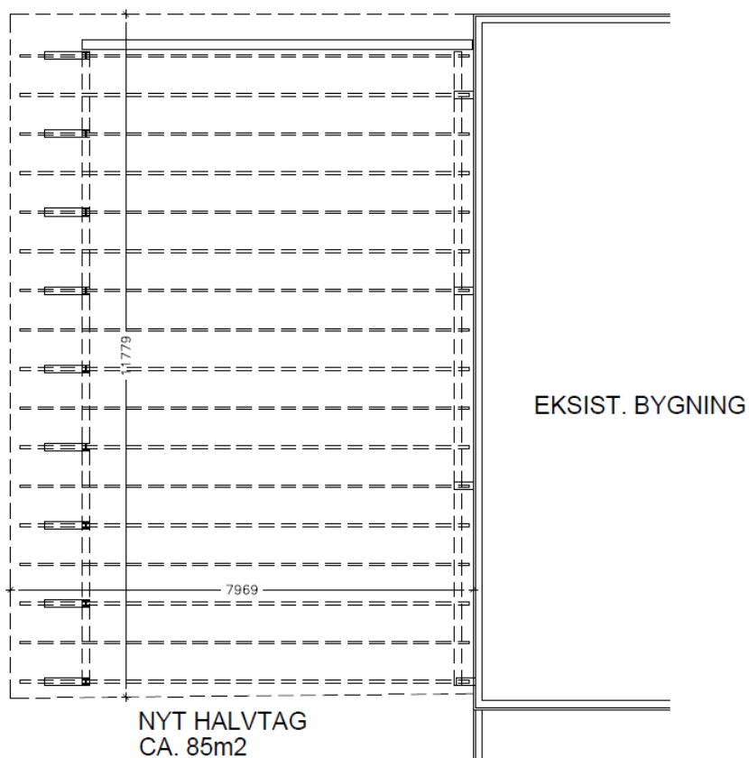
Plantegning fra ansøgning
