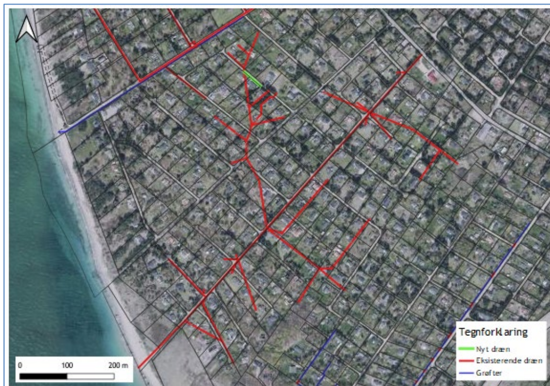
Figur 2 - Kort over afvandingssystemet.
