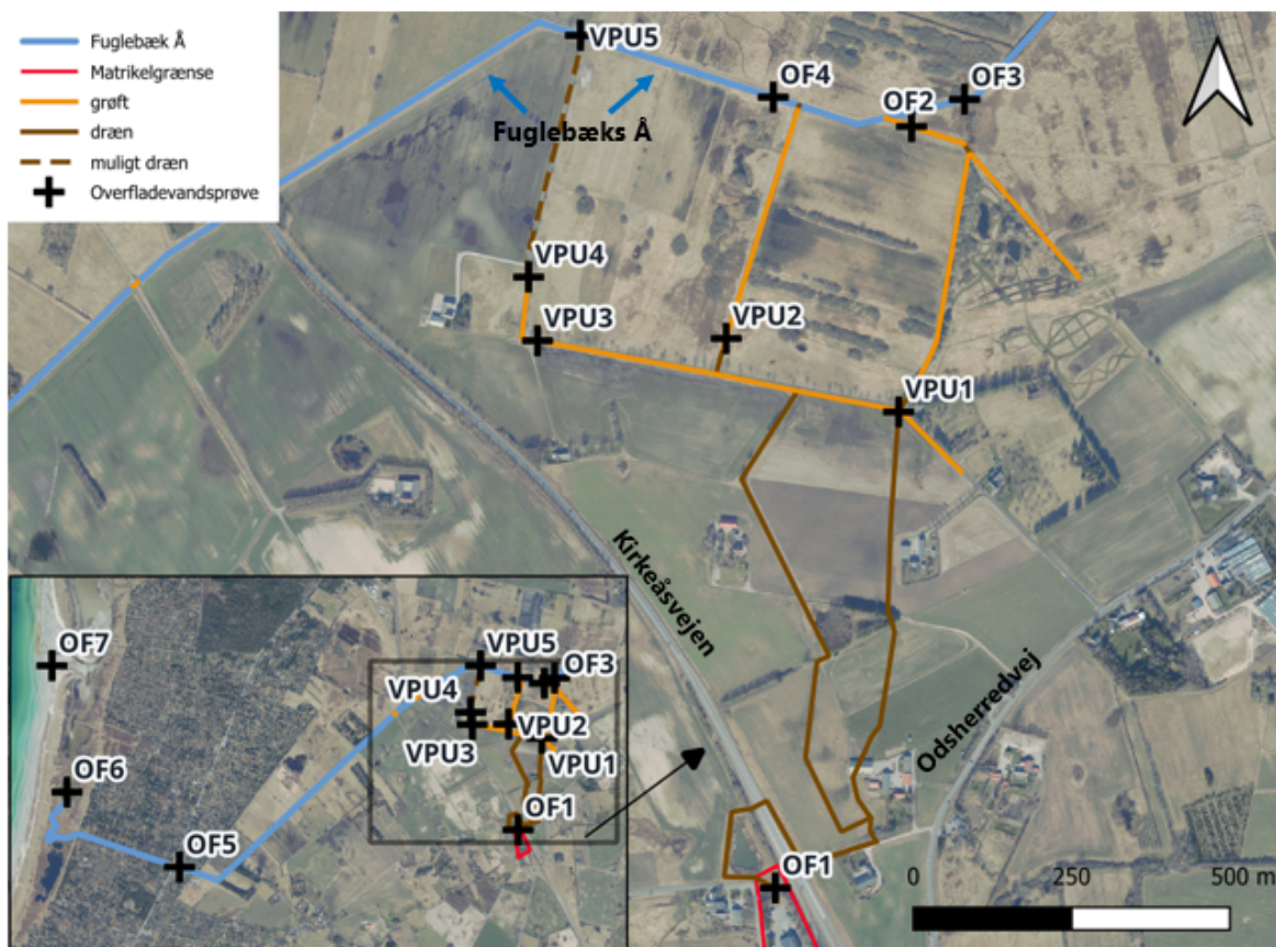
Figur 1: Placering af dræn og grøfter, nedstrøms Nørremarksvej 13
