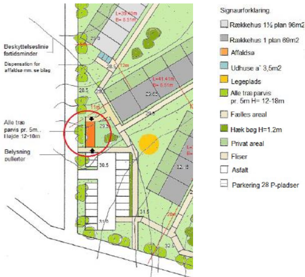
Figur 2. Udsnit af situationsplanen fra ansøgningen.
