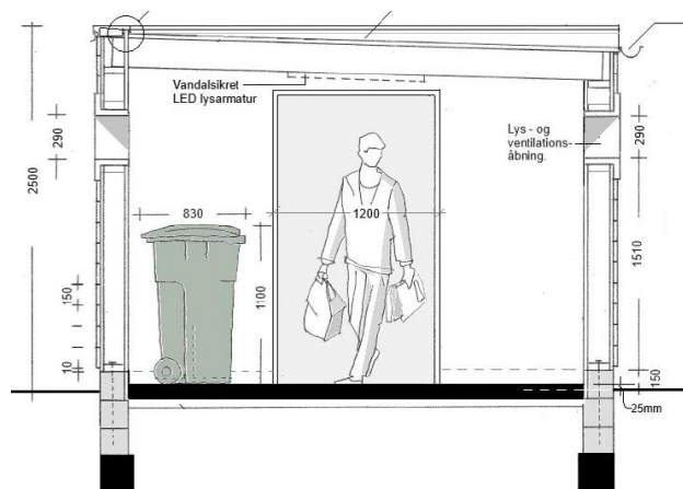
Figur 5. Snit (fra ansøgningsmaterialet).
