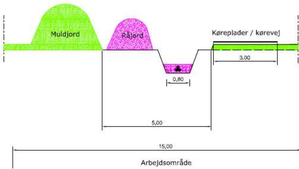
Figur 1: Skitsering af kabelgravearbejdet.
