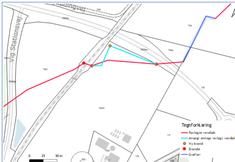
Figur 1 – Oversigtskort med eksisterende drænløb og omlagt forløb.
