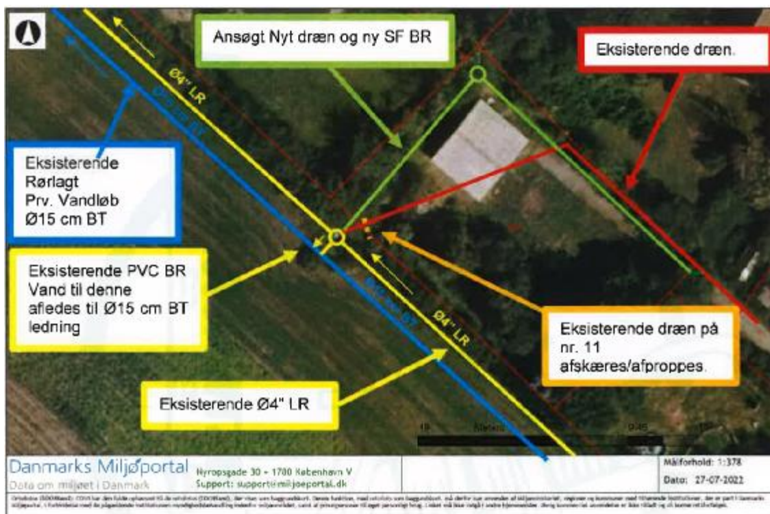
Figur 1 - Kort med det nuværende forløb af drænet på Klintvej 11, 4500 Nykøbing Sj. vist med rødt samt det nye forløb af drænet med grønt. Eksisterende rørlagt vandløb er vist med blå og eksisterende dræn langs marken med gult.
