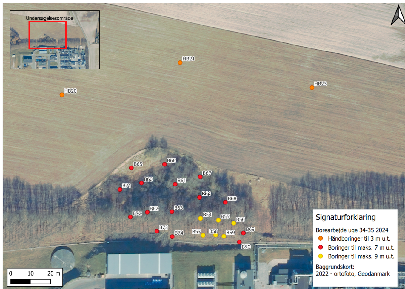
Placering af borerne på matrikel 7o Lumsås By, Højby
