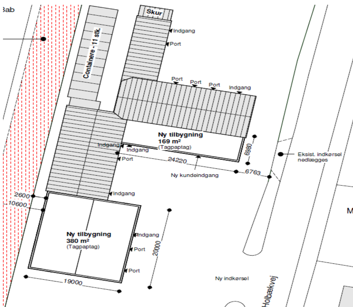
Situationsplan med eksisterende bygninger og de ansøgte tilbygninger.
