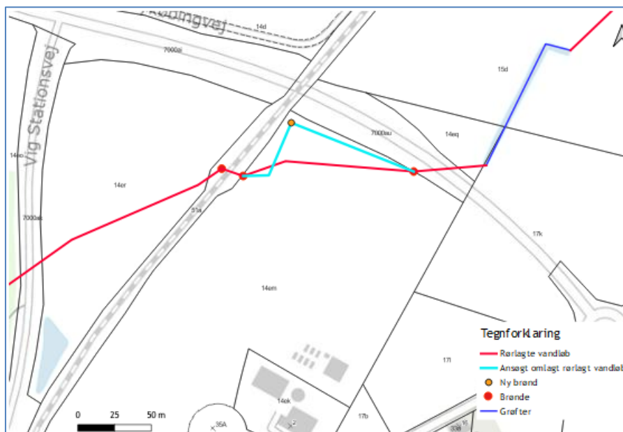
Figur 1 – Oversigtskort med eksisterende dræneløb og omlagt forløb.
